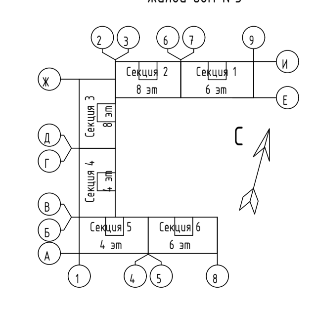
Компоновочная схема Жилой дом №3
